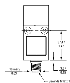
Gehäusetyp 'D'
